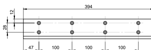
Kątownik montażowy siłownika AC633 Dla wersji montażowych siłownika po stronie Push i montażu na ścianie
