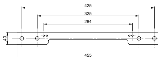
Płyta montażowa AC632 W przypadku braku odpowiedniej płaszczyzny montażowej dla szyny
